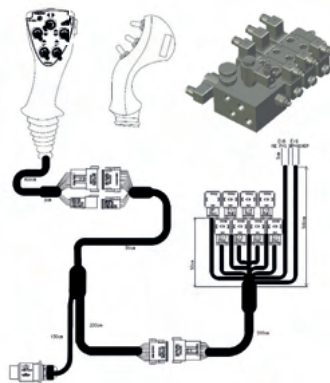
Kits de distribution hydraulique
