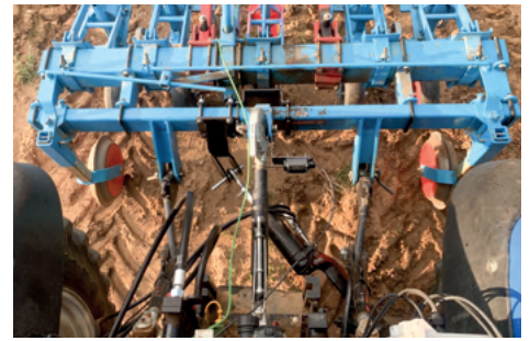
Attelage 4ème point
