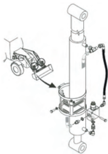
Kits clapets de sécurité
