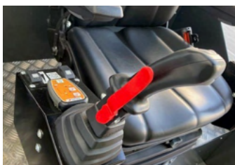
Joystick Detect
