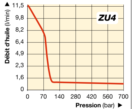
COURBE DE DÉBIT
