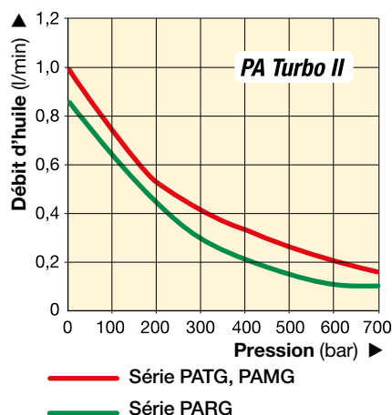
COURBE DE DÉBIT
